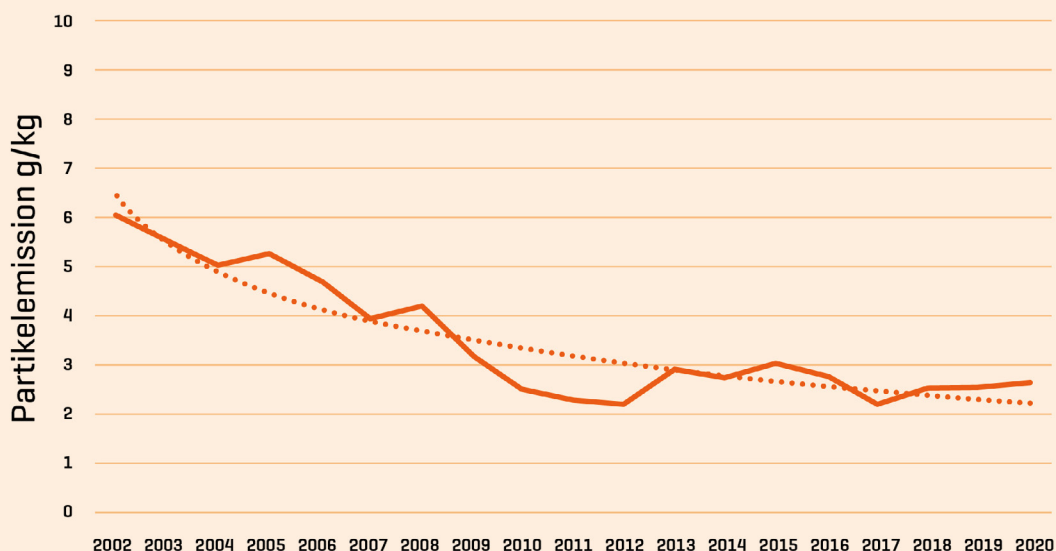
Udvikling i partikelemission for brændeovne testet af Teknologisk Institut 2002-2020
